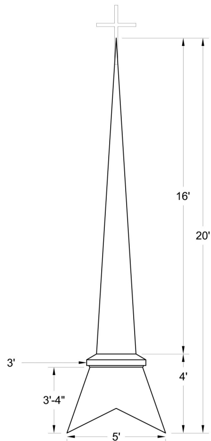
ELEVATION Scale: 1/4" = 1'-0"
