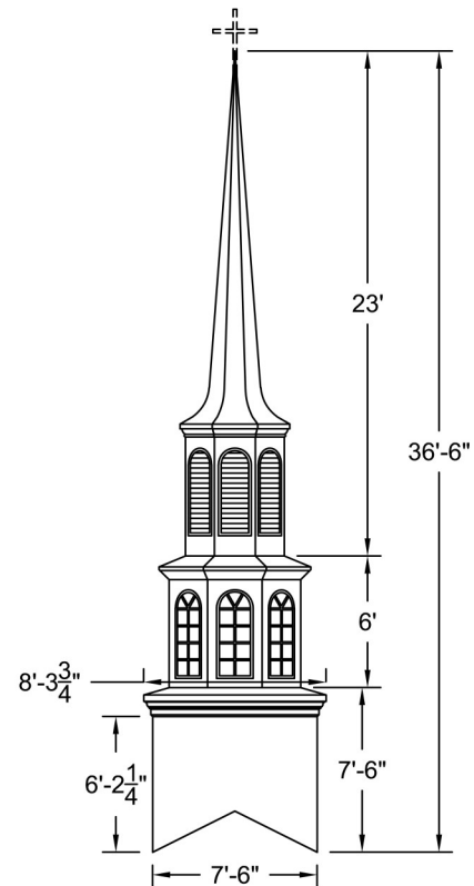
ELEVATION Scale: 1/8" = 1'-0"
