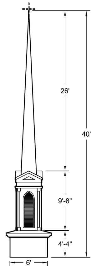
ELEVATION Scale: 1/8" = 1'-0"
