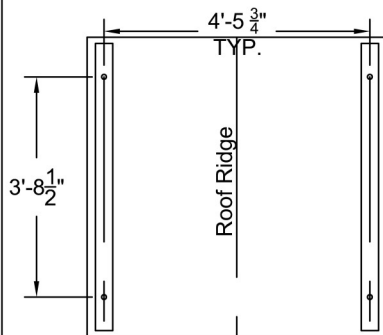
Plan View A-A Scale: 3/8" = 1'-0"
