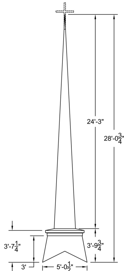
ELEVATION Scale: 3/16" = 1'-0"
