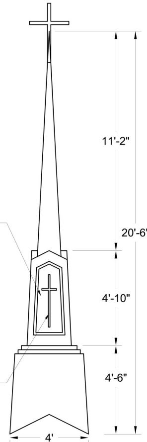
ELEVATION Scale: 1/4" = 1'-0"
