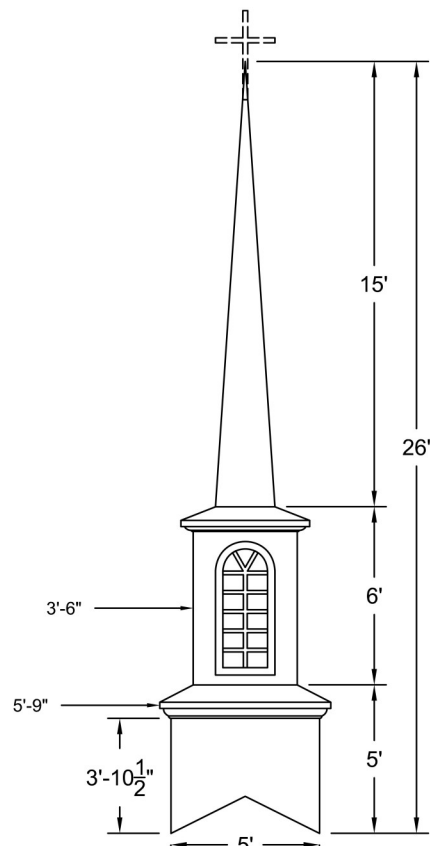
ELEVATION Scale: 3/16" = 1'-0"
