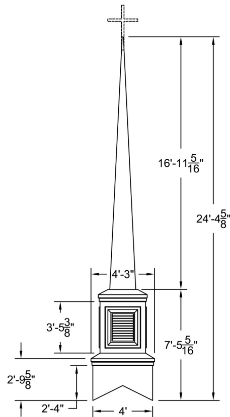
ELEVATION Scale: 3/16" = 1'-0"
