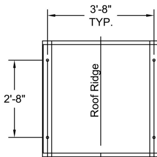
Plan View A-A Scale: 3/8" = 1'-0"
