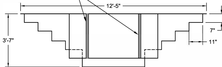
Front View Scale: 3/8" = 1'-0"
