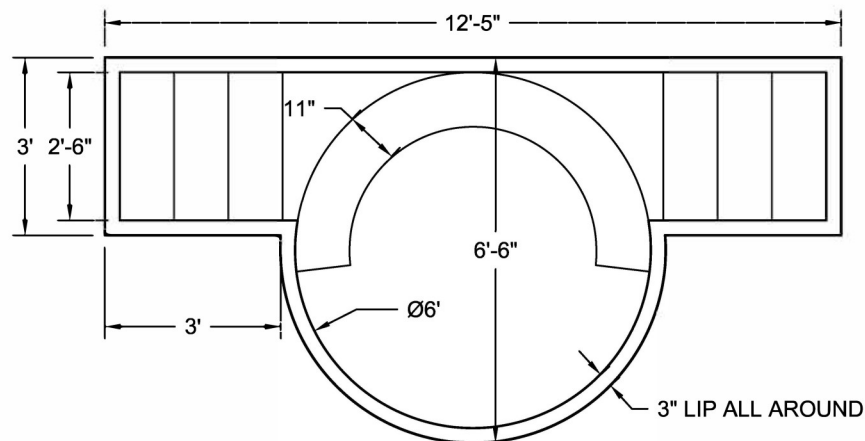
TOP VIEW Scale: 3/8" = 1'-0"
