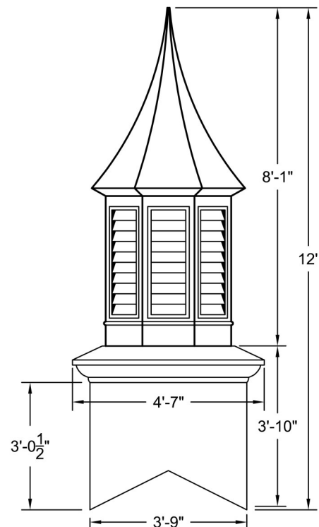
ELEVATION Scale: 3/8" = 1'-0"
