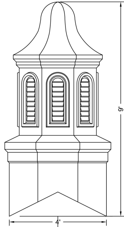
ELEVATION Scale: 1/4" = 1'-0"
