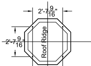
Plan View A-A Scale: 1/4" = 1'-0"
