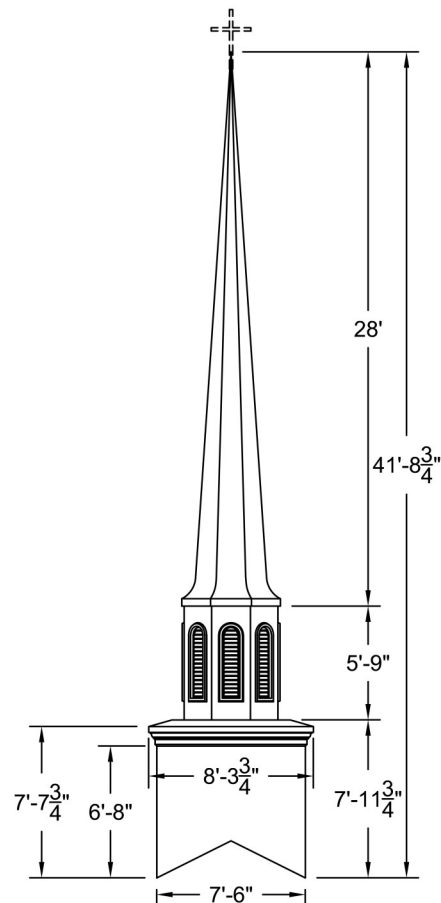
ELEVATION Scale: 1/8" = 1'-0"
