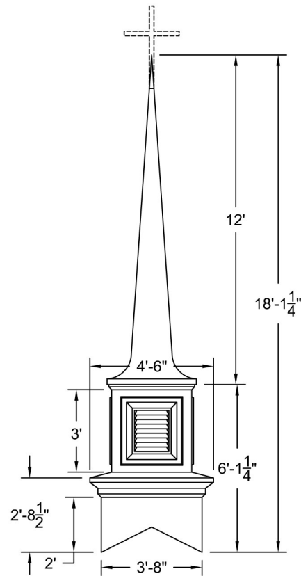
ELEVATION Scale: 1/4" = 1'-0"
