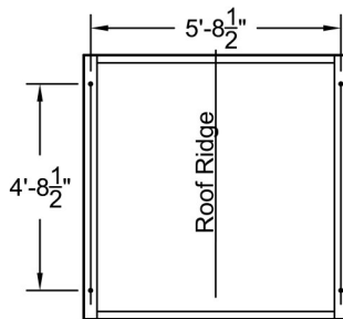
Plan View A-A Scale: 1/4" = 1'-0"
