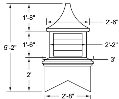
ELEVATION Scale: 3/8" = 1'-0"
