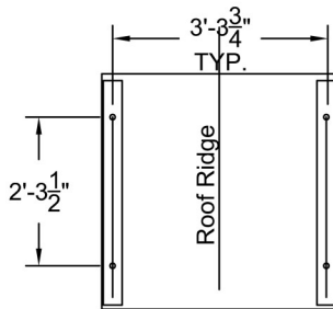
Plan View A-A Scale: 3/8" = 1'-0"
