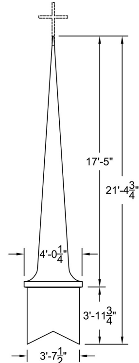
ELEVATION Scale: 3/16" = 1'-0"
