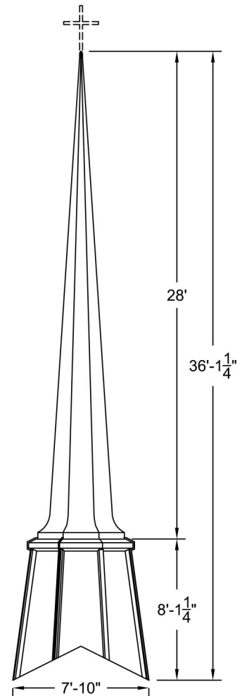
ELEVATION Scale: 5/32" = 1'-0"
