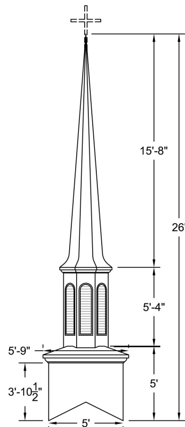
ELEVATION Scale: 3/16" = 1'-0"
