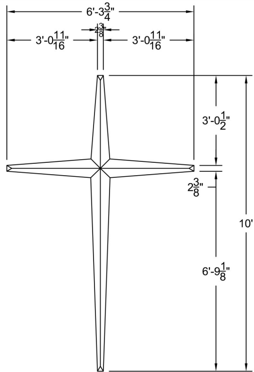
Front View Scale: 3/8" = 1'-0"
