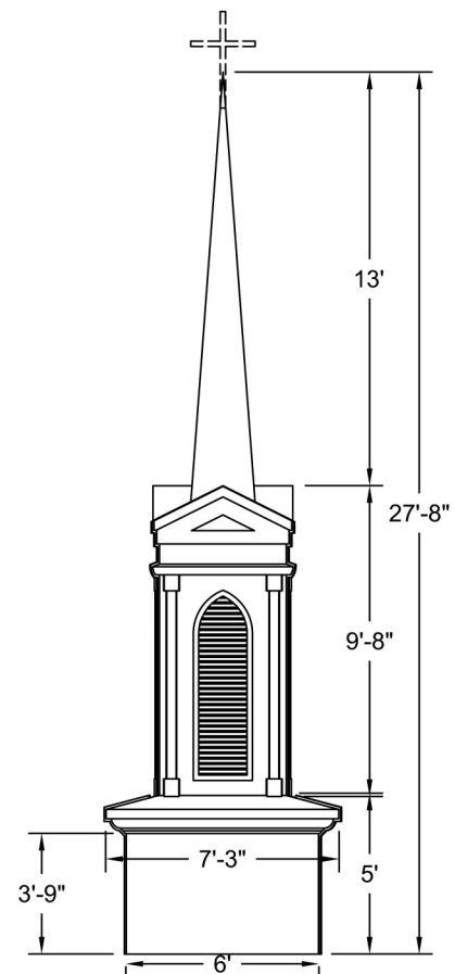
ELEVATION Scale: 3/16" = 1'-0"
