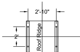
Plan View A-A Scale: 1/4" = 1'-0"
