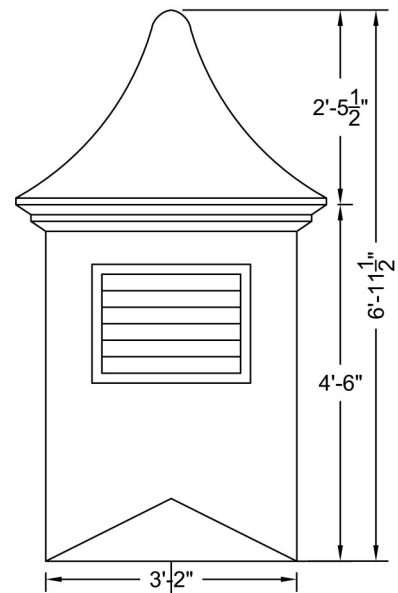
ELEVATION Scale: 1/4" = 1'-0"
