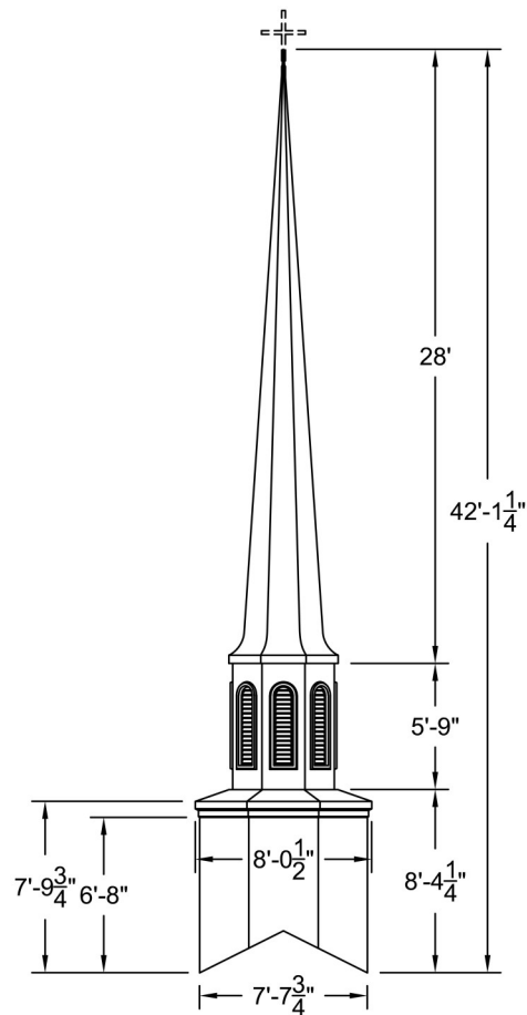
ELEVATION Scale: 1/8" = 1'-0"
