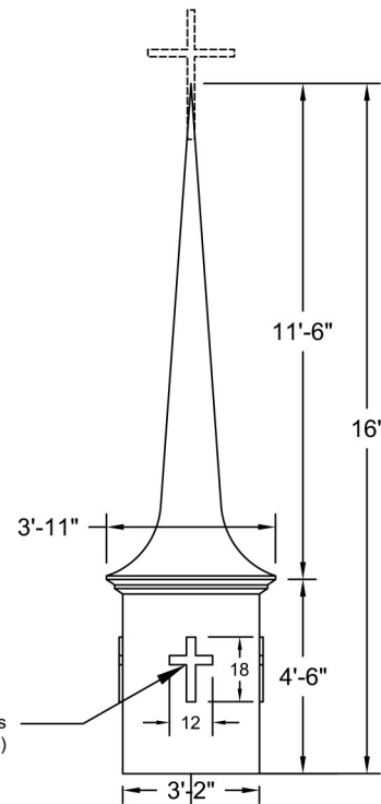
ELEVATION Scale: 1/4" = 1'-0"
