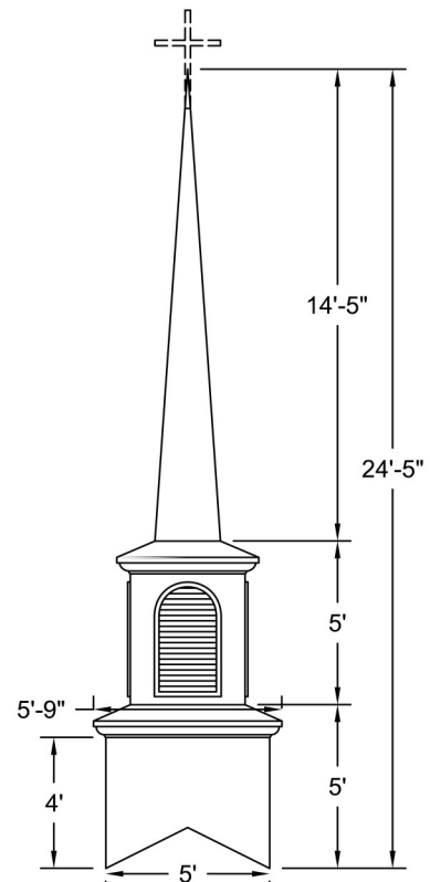
ELEVATION Scale: 3/16" = 1'-0"
