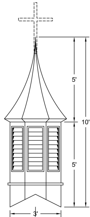
ELEVATION Scale: 3/8" = 1'-0"
