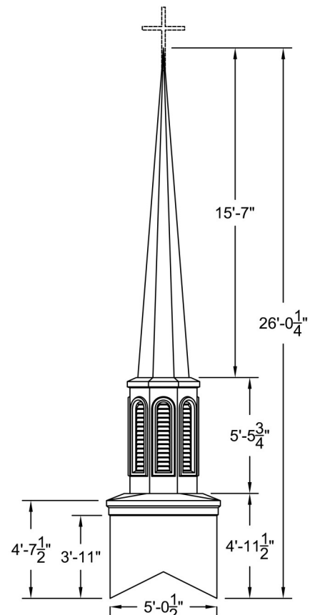
ELEVATION Scale: 3/16" = 1'-0"
