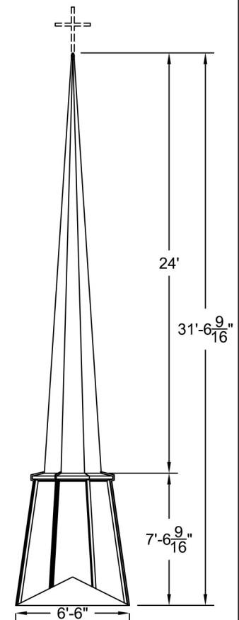
ELEVATION Scale: 5/32" = 1'-0"
