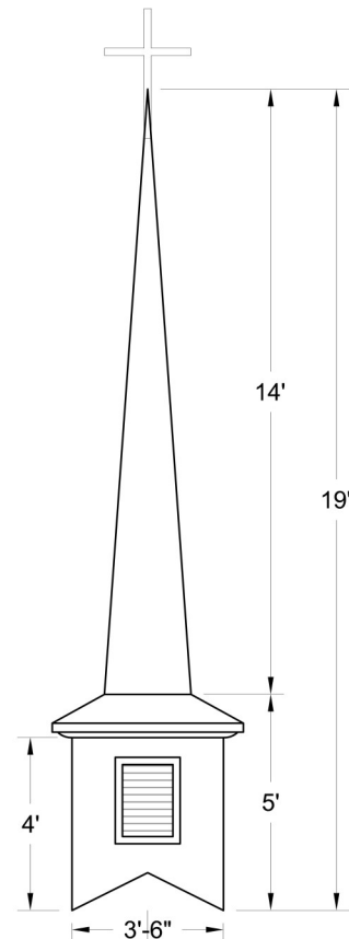
ELEVATION Scale: 1/4" = 1'-0"
