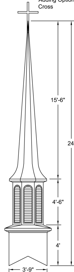
ELEVATION Scale: 1/4" = 1'-0"
