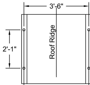
Plan View A-A Scale: 3/8" = 1'-0"
