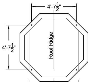
Plan View A-A Scale: 1/4" = 1'-0"
