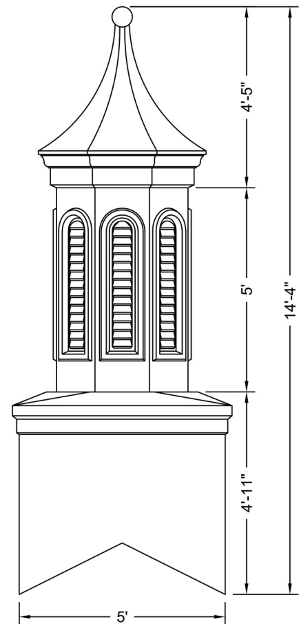
ELEVATION Scale: 3/8" = 1'-0"
