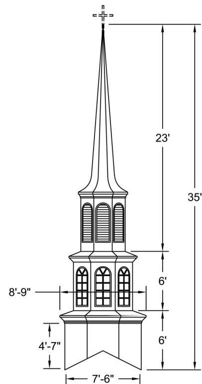
ELEVATION Scale: 1/8" = 1'-0"
