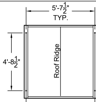
Plan View A-A Scale: 1/4" = 1'-0"
