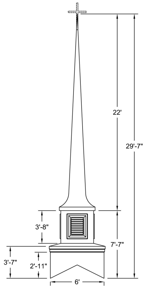
ELEVATION Scale: 3/16" = 1'-0"
