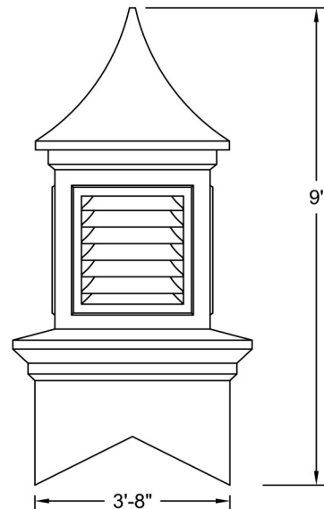
ELEVATION Scale: 3/8" = 1'-0"
