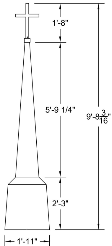
ELEVATION Scale: 1/2" = 1'-0"
