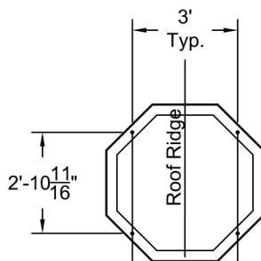
Plan View A-A Scale: 1/4" = 1'-0"
