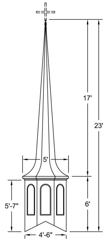
ELEVATION Scale: 3/16" = 1'-0"
