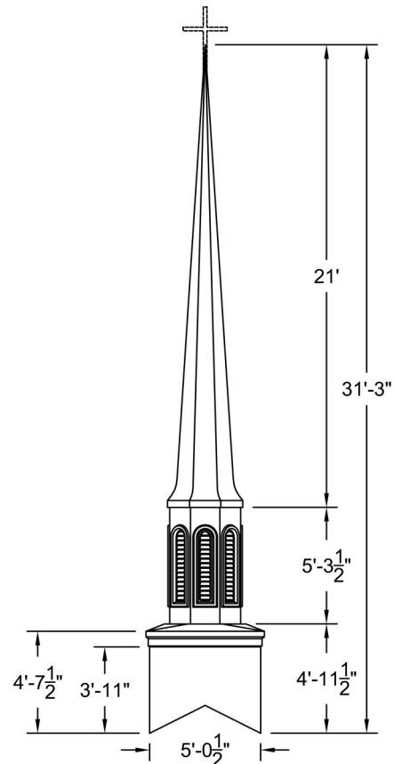
ELEVATION Scale: 5/32" = 1'-0"
