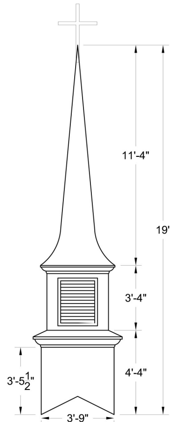
ELEVATION Scale: 1/4" = 1'-0"
