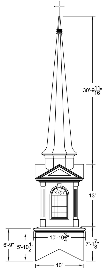
ELEVATION Scale: 1/8" = 1'-0"
