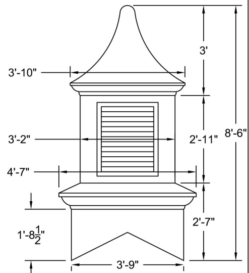
ELEVATION Scale: 3/8" = 1'-0"
