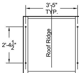
Plan View A-A Scale: 3/8" = 1'-0"
