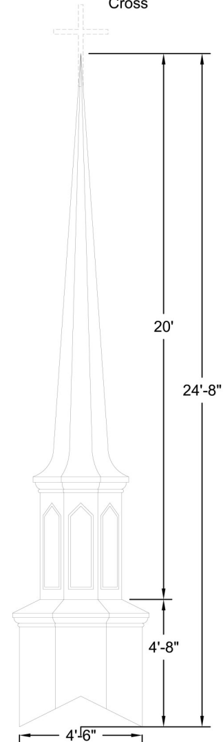
ELEVATION Scale: 1/4" = 1'-0"
