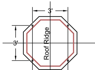
Plan View A-A Scale: 1/4" = 1'-0"
