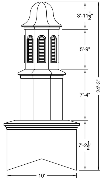
ELEVATION Scale: 1/4" = 1'-0"
