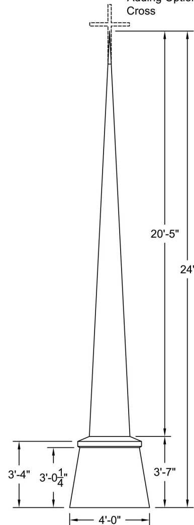
ELEVATION Scale: 1/4" = 1'-0"
