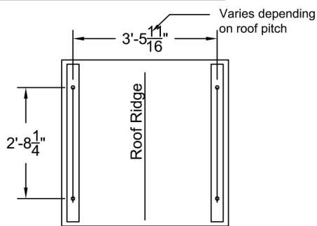
Plan View A-A Scale: 3/8" = 1'-0"
