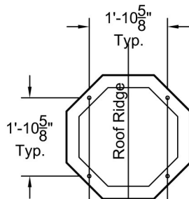
Plan View A-A Scale: 3/8" = 1'-0"
