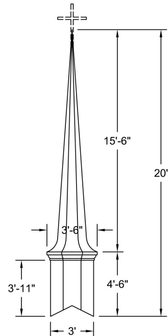
ELEVATION Scale: 3/16" = 1'-0"
