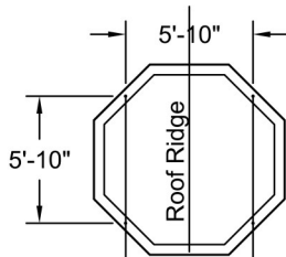
Plan View A-A Scale: 1/8" = 1'-0"
