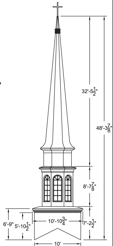
ELEVATION Scale: 1/8" = 1'-0"
