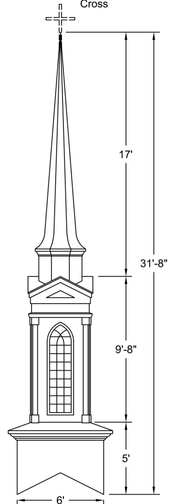
ELEVATION
