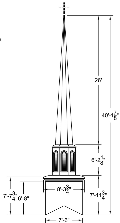
ELEVATION Scale: 1/8" = 1'-0"
